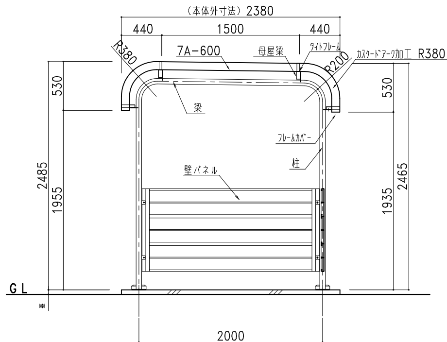
側面断面図
