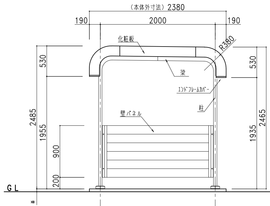
側面図
