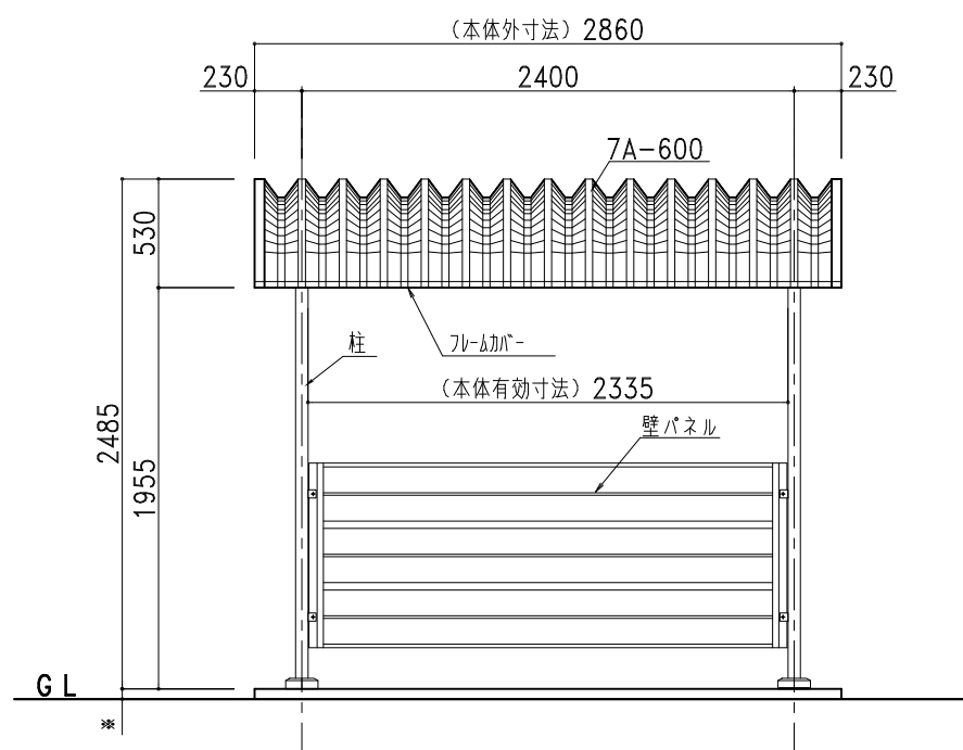
正面义
