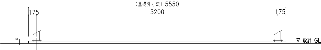
基礎正面図 1/40
