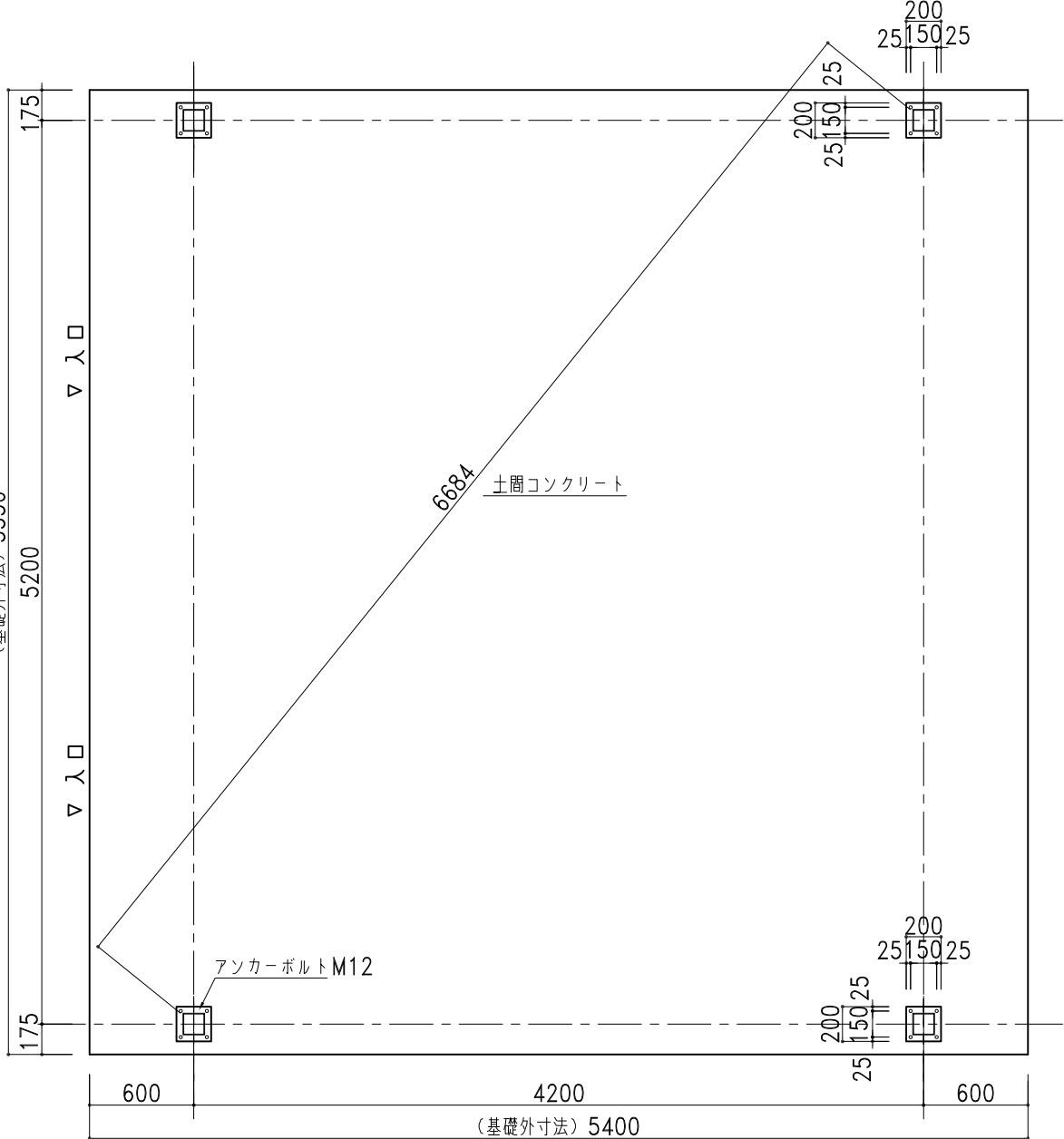
基礎伏図 1/40
