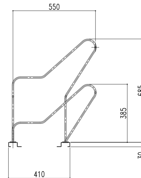
断面側面図
