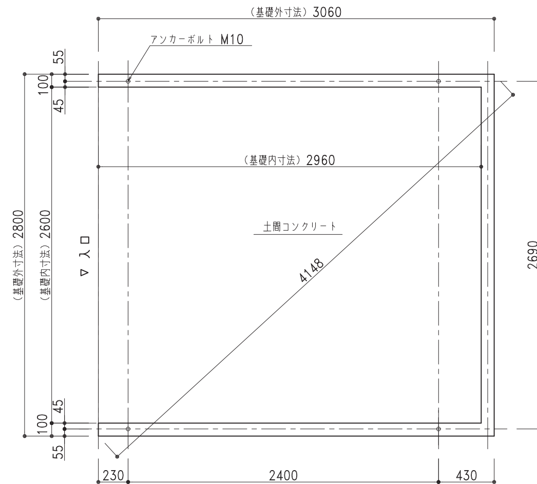
基礎伏図 1/30
