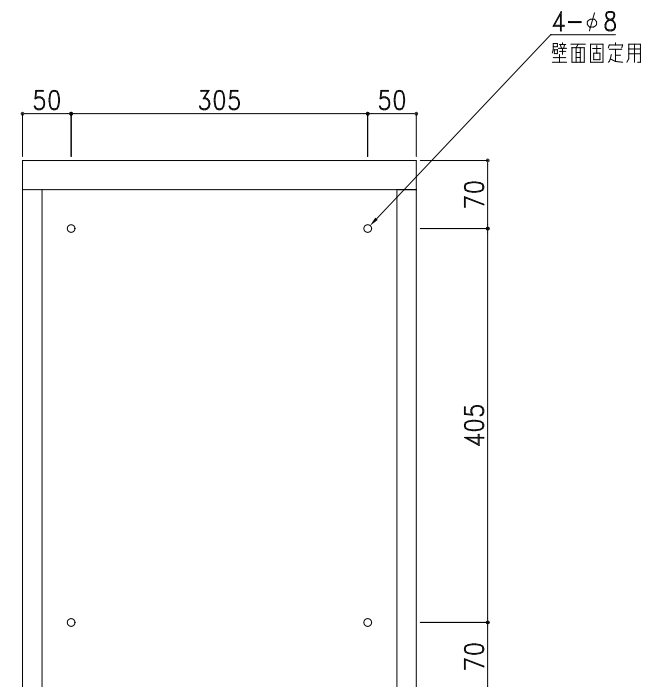
背面図
