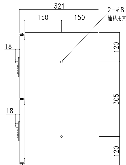
右側面図
