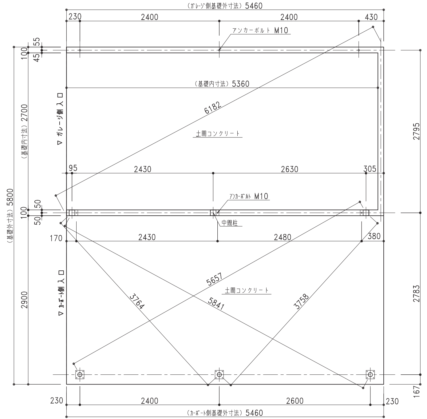
基礎伏図 1/40
