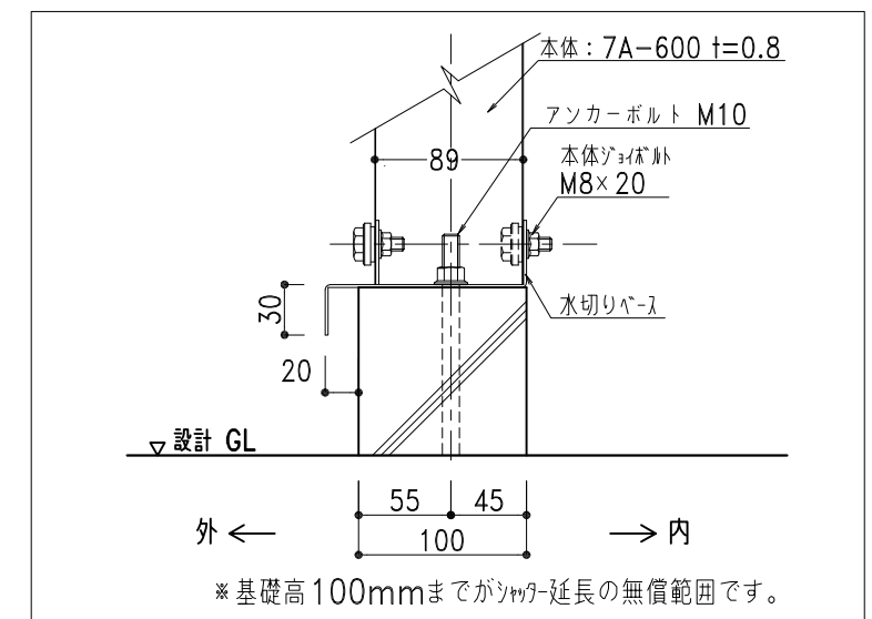
ベ-ス取付図 1/5
