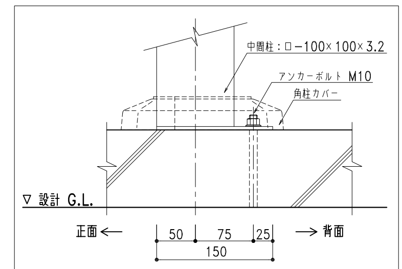
中間柱取付図 1/5
