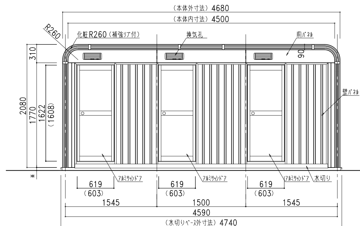
正面図
