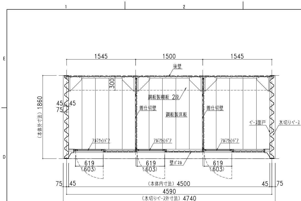
平面图
