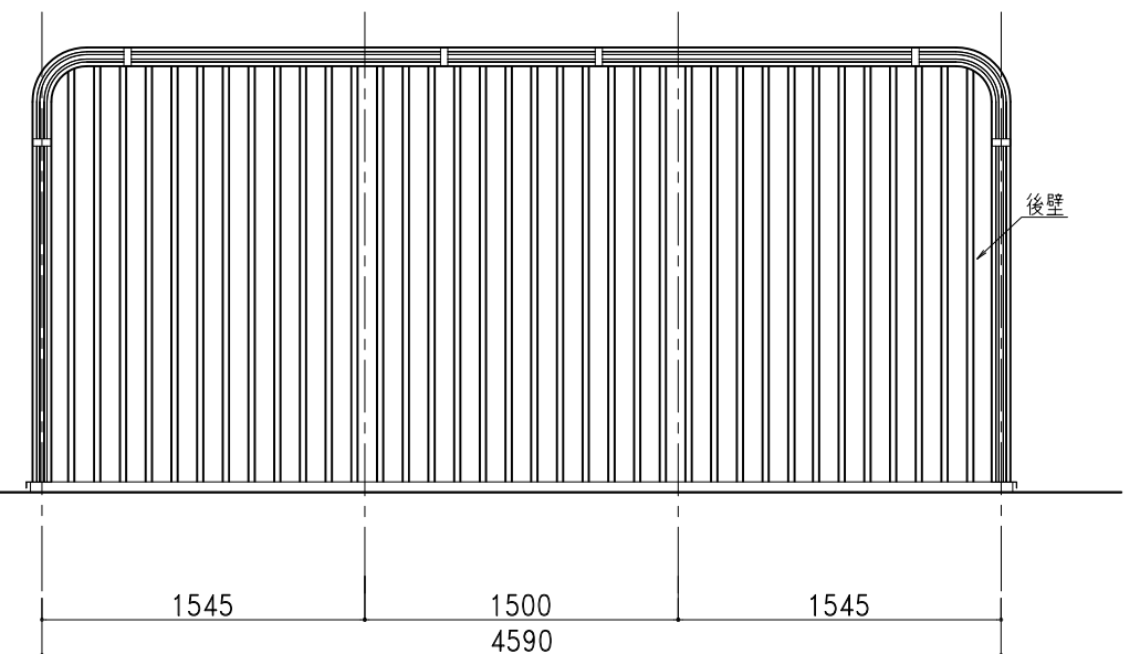
背面図
