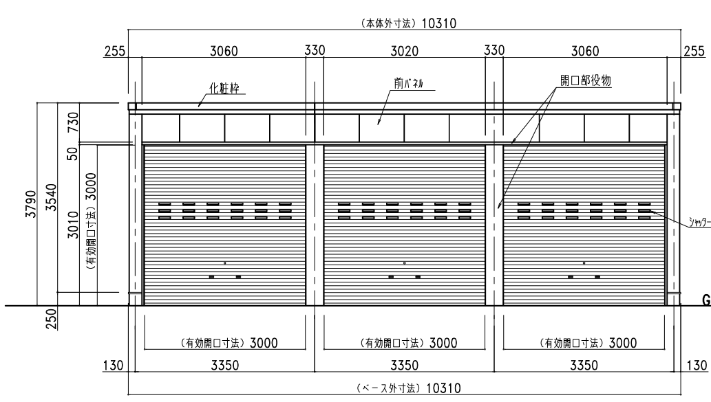
正面図
