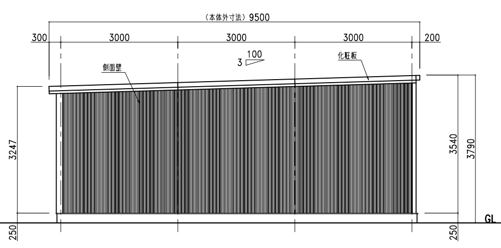
右側面図
