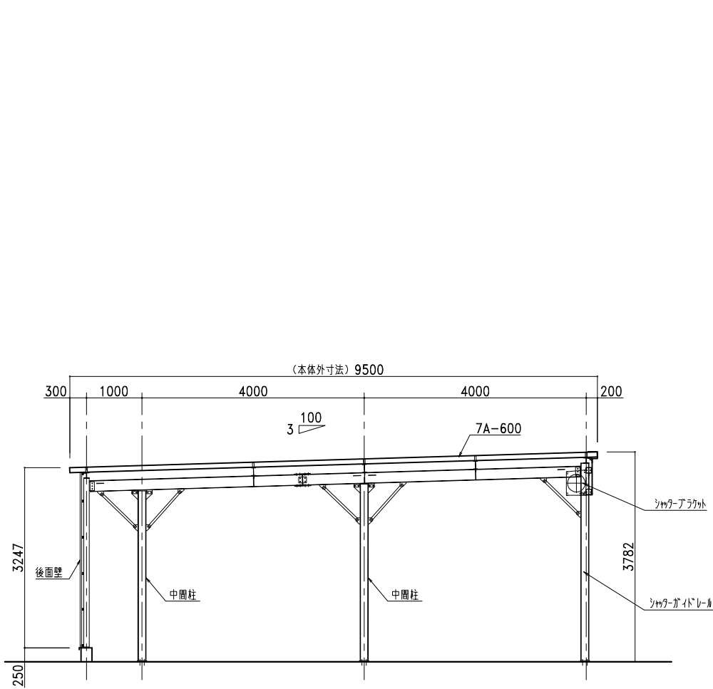
連棟部梁構造図
