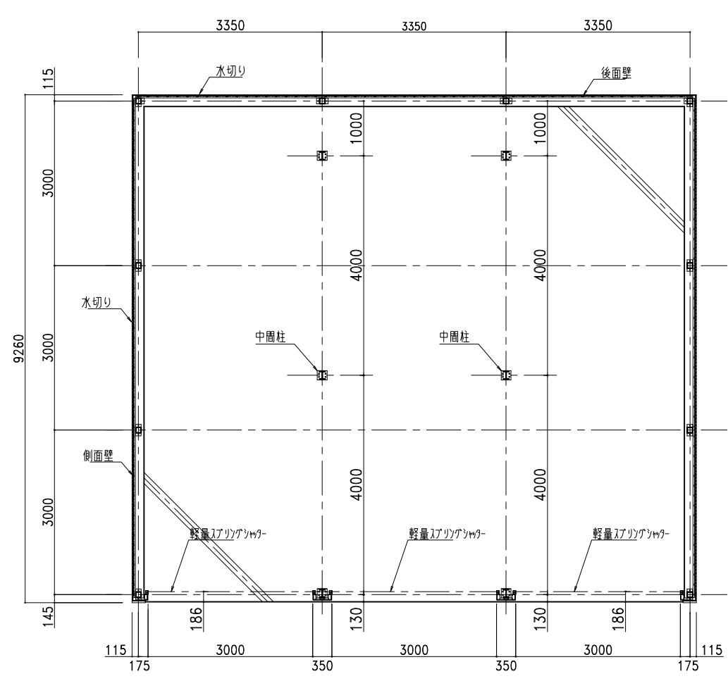
平面図
