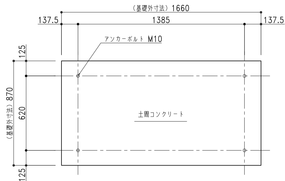
基礎伏図 1/20 ※○は、アソカー位置を示します。
