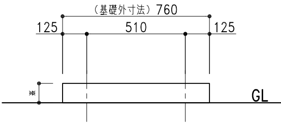
基礎側面図 1/20
