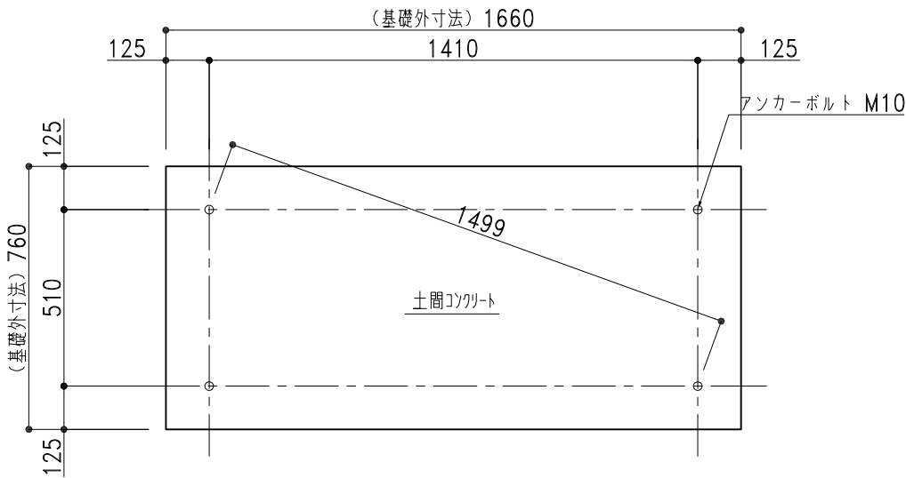
基礎伏図 1/20 ※○は、アンカー位置を示します。
