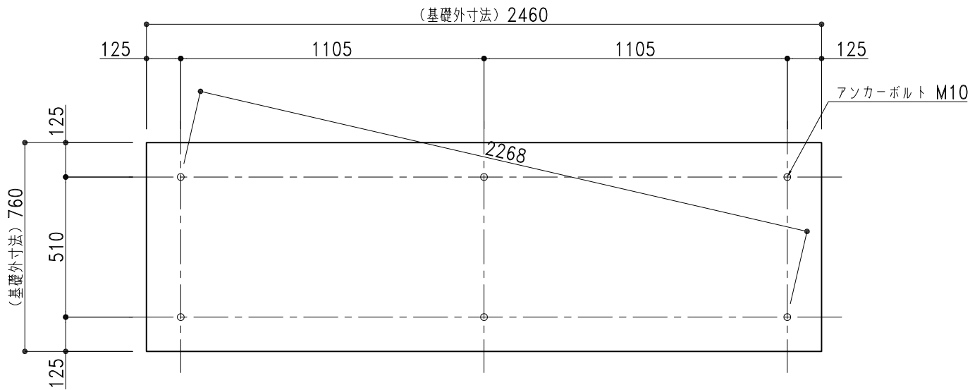
基礎伏図 1/20 ※○は、アンカー位置を示します。
