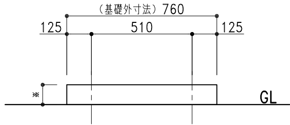
基礎側面図 1/20
