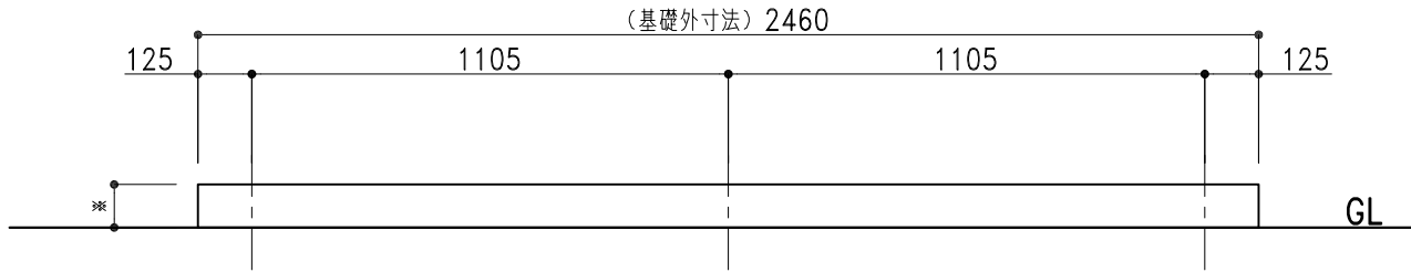
基礎正面図 1/20
