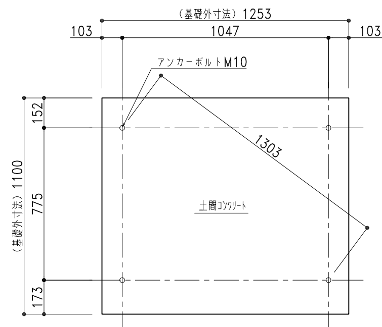
基礎伏図 1/20 ※○は、アソカー位置を示します。
