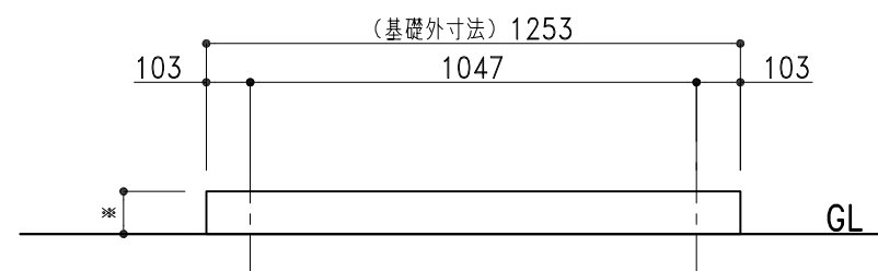
基礎正面図 1/20
