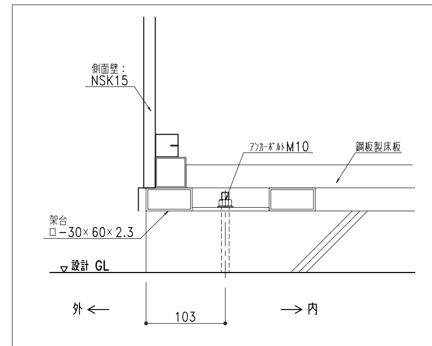
基礎納まり図 1/5
