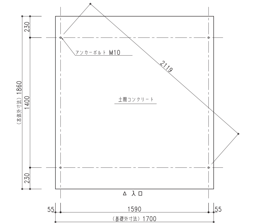
基礎伏図 1/20 ※○は、アンカー位置を示します。
