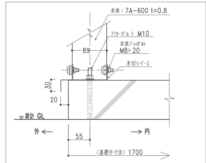
水切りベース納まり図 1/5
